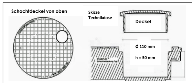
Skizze Swiss-Edition DN 600 mit CH-Modulrahmen – Abmessungen ca. Angaben in mm
