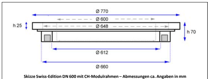
Skizze Swiss-Edition DN 600 mit CH-Modulrahmen – Abmessungen ca. Angaben in mm
