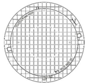
Skizze Swiss-Edition DN 600 CH-Modulrahmen mit Deckel OG Ansicht von oben
